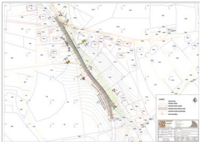
Območje in situacija obnove regionalne ceste in izgradnje pločnika z JR
